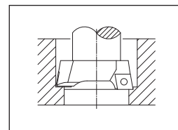
Due taglienti su diametri diversi
