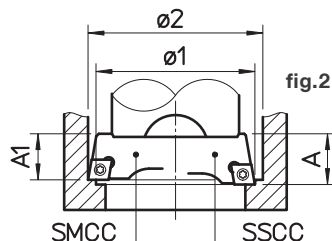
fig. 2 con un seggio SSCC ed un seggio SMCC disallineato e su un diverso diametro per operazioni di sgrossatura con alte profondità di passata.
