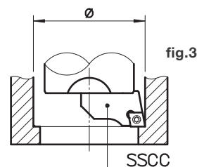
fig.3 con un solo seggio per operazioni di sgrossatura leggera o semifinitura.
