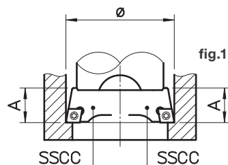
fig.1 con due seggi SSCC allineati e sullo stesso diametro per operazioni di sgrossatura con forti avanzamenti.
