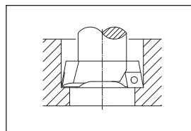
Due taglienti sullo stesso diametro
