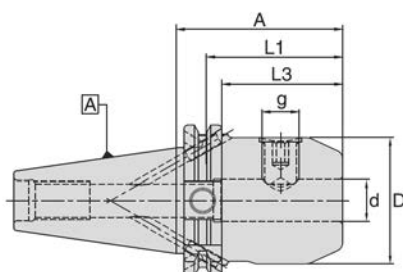
Mandrino SK40 per fresa a candela / Weldon Portaherramientas SK40 para fresa tipo endmill / Weldon
