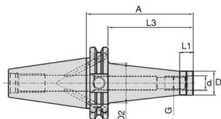
Mandrino SK40 per fresa con attacco filettato Portaherramientas SK40 para fresa atornillable
