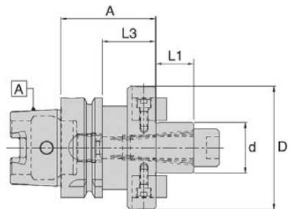
Mandrino HSK-A100 per fresa a manicotto Portaherramienta HSK-A100 para fresa de planeado
