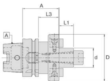
Mandrino HSK-A63 per fresa a manicotto Portaherramienta HSK-A63 para fresa de planeado
